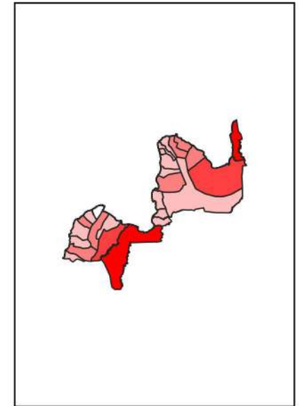
HAZARD INDEX
